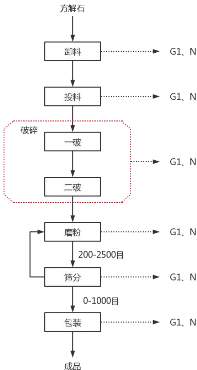
图 2-2 项目生产工艺流程及产污节点图
