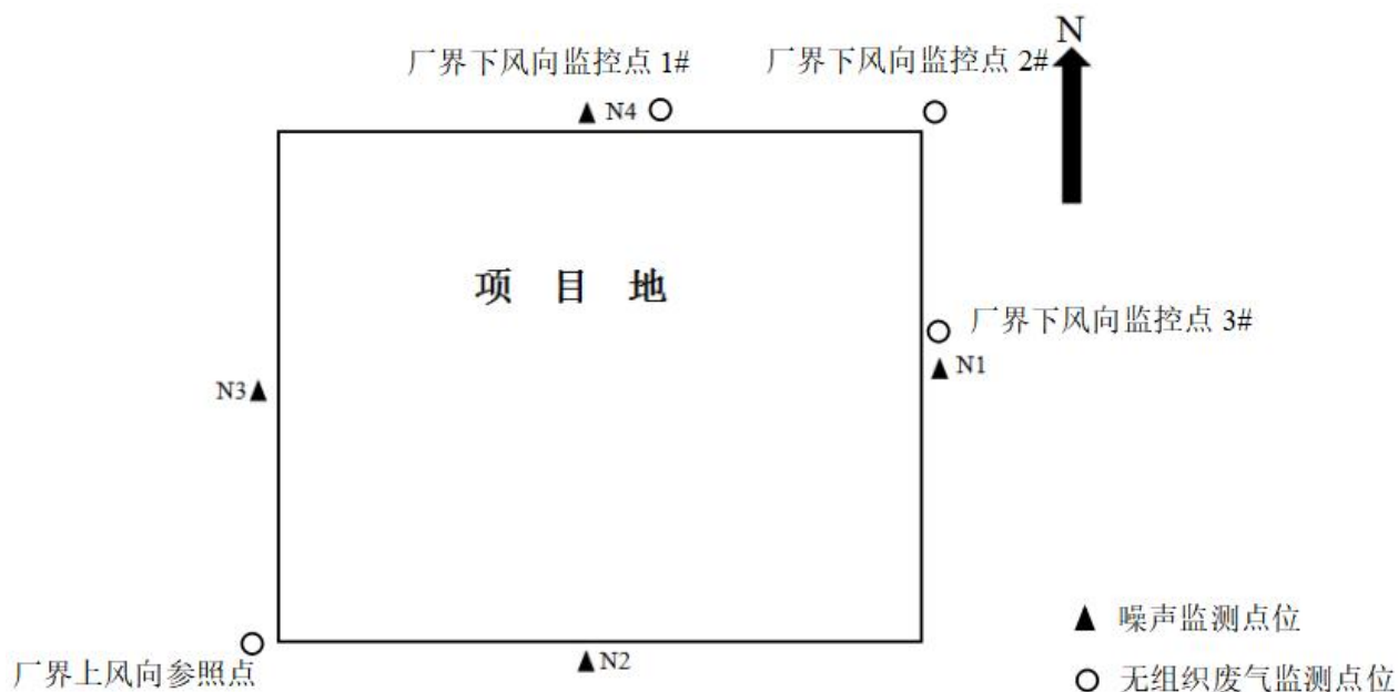
图 6-1 2024 年 1 月 3 日噪声及无组织废气监测点位示意图
