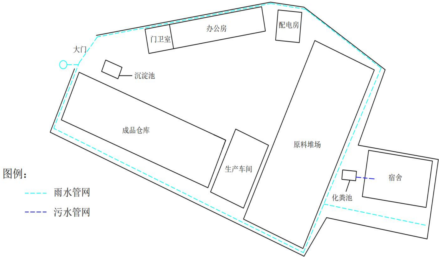
附图 2：雨污水管网图
